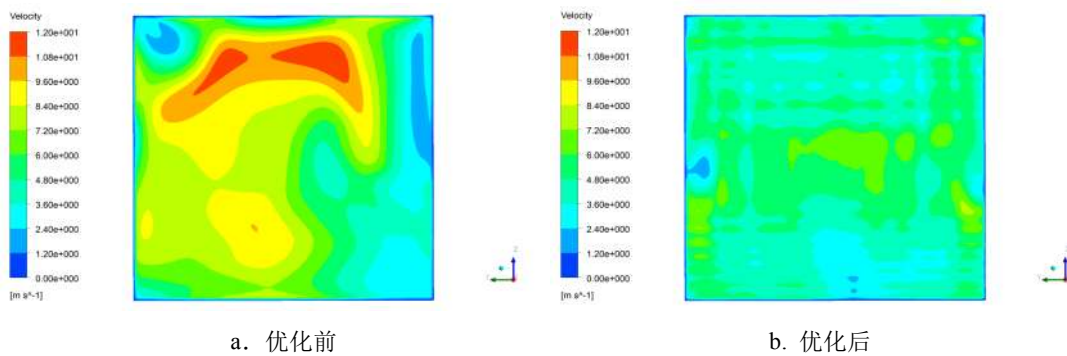
图 18 脱硫塔出口烟道除雾器上游断面速度分布
