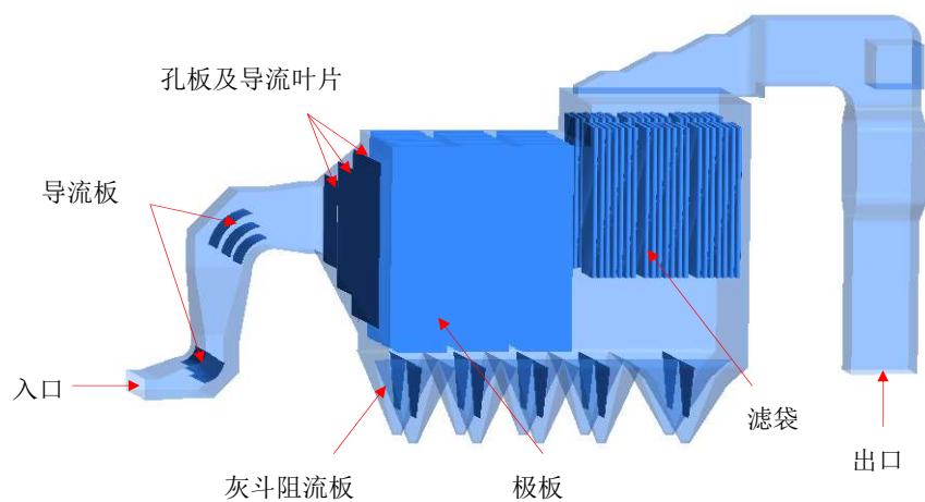
图 7 电袋复合除尘器 CFD 模型
