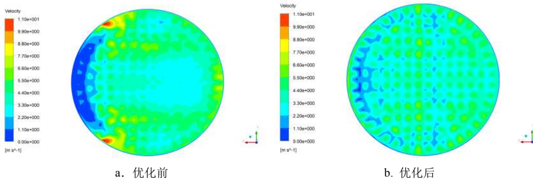
图 17 脱硫塔内首层喷淋层上游断面速度分布
