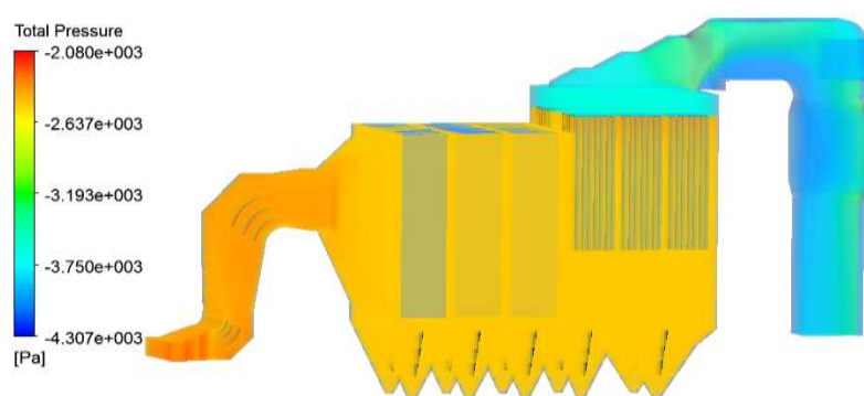
图 9 电袋复合除尘器压力分布
