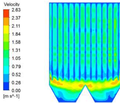
图 10 电袋复合除尘器电场前断面速度分布
