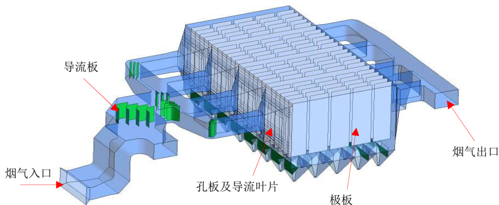
图3 电除尘器 CFD 模型
