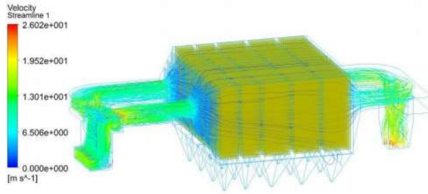
图 5 电除尘器内部流线图
