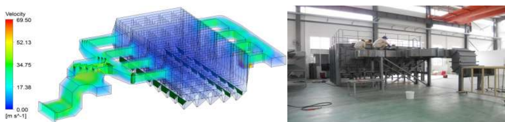
图4 电除尘器流场数值模拟和物模试验
