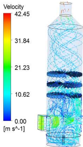
图 19 麻石脱硫塔内烟气流线
