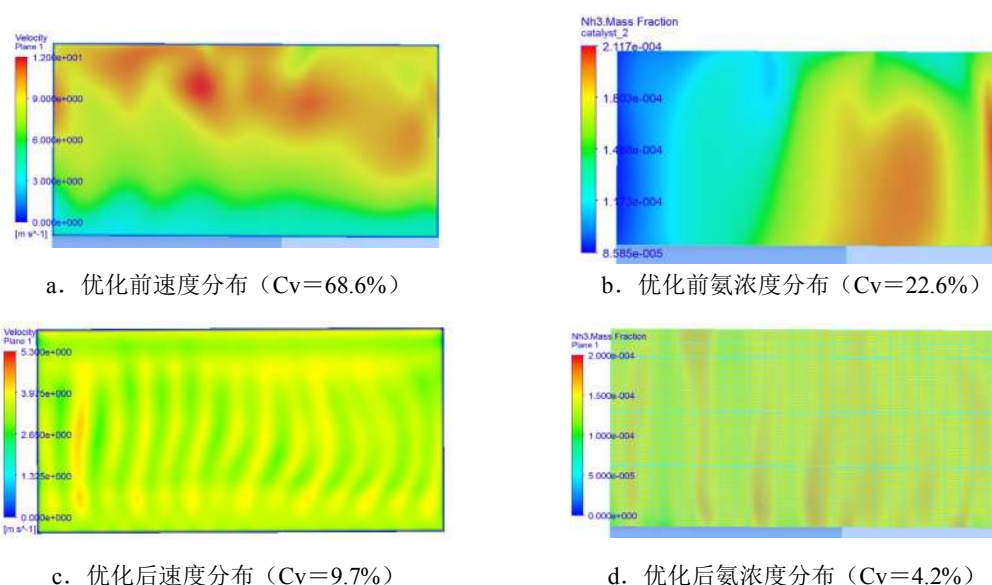
图 14 优化前后催化剂入口断面速度分布和浓度分布对比
