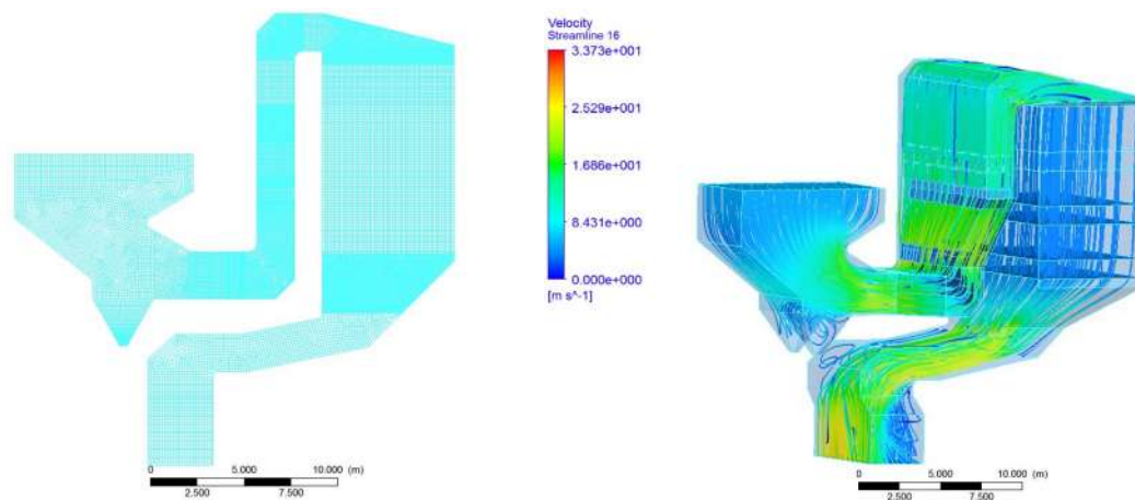
图 13 SCR 脱硝装置 CFD 模型网格划分及数值模拟结果
