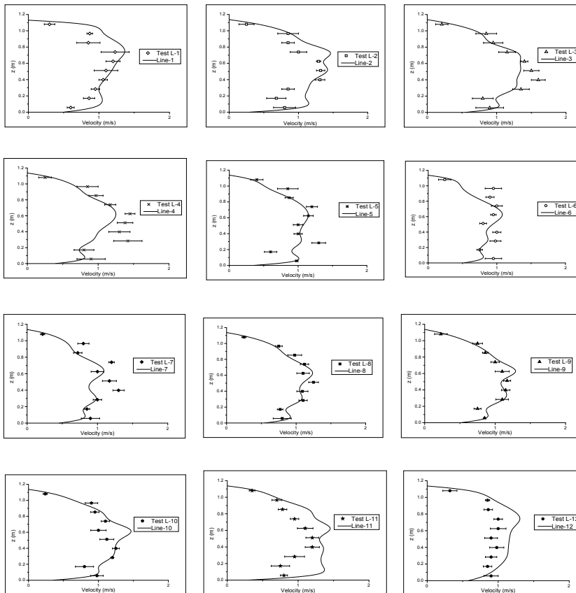
图 6 电除尘器电场第一断面气流分布数值模拟和试验对比结果
