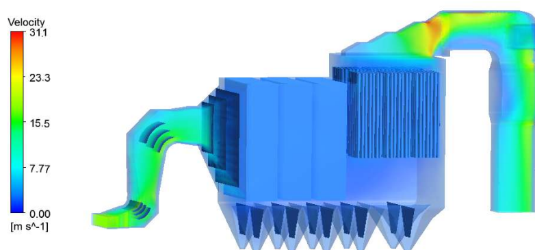
图 8 电袋复合除尘器速度分布
