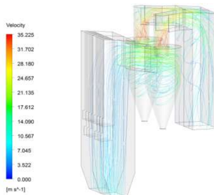
图 11 CFB 锅炉内部流场
