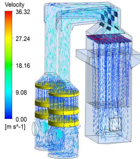
图 20 工业炉窑湿法电除尘器内烟气流线
